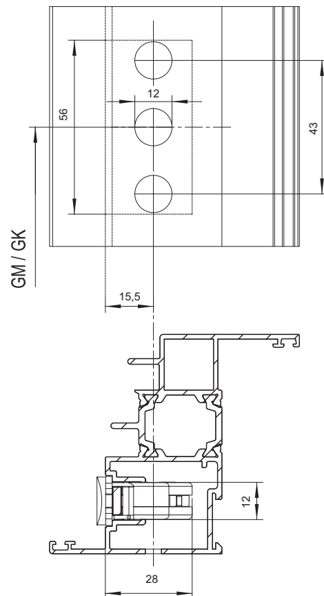
Maßzeichnung "Getriebeschloss"
