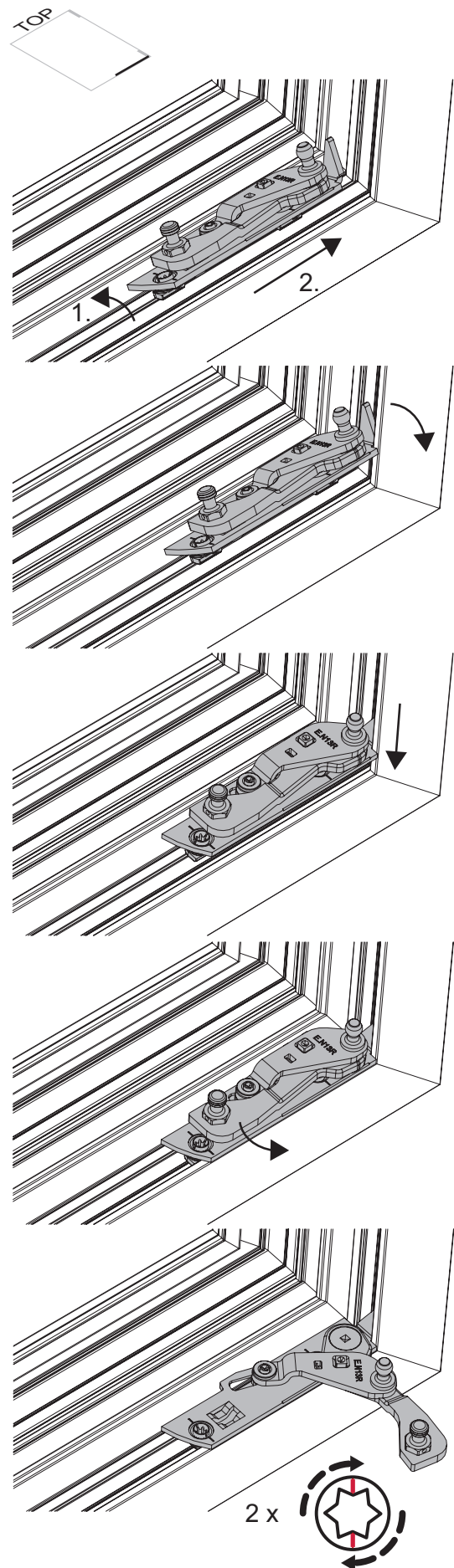
Ecklager montieren
