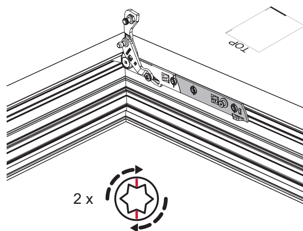
Rahmenanbindung montieren
