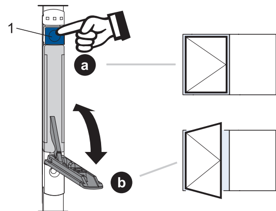
Funktionstest Stulpfenster
