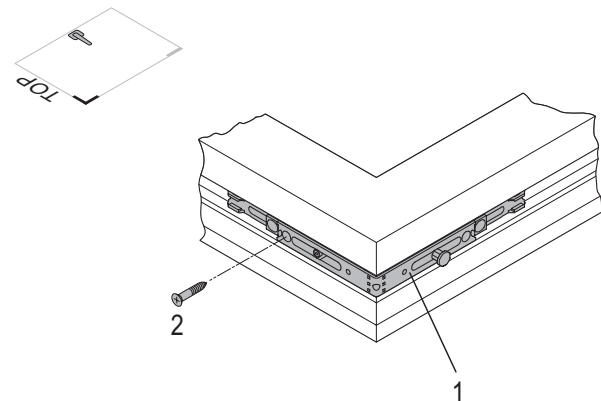
Eckumlenkung E1.SE
